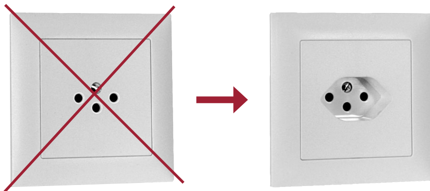
Steckdose Typ 12 Prise type 12 Presa tipo 12
